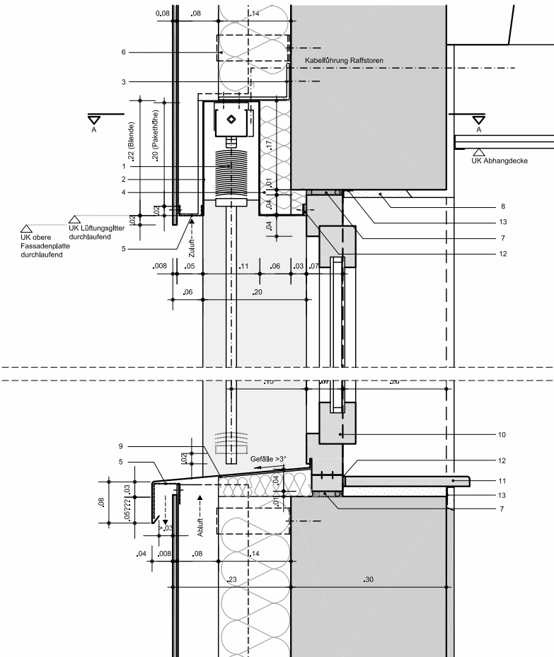
Detail Thermische Sanierung Fassade
